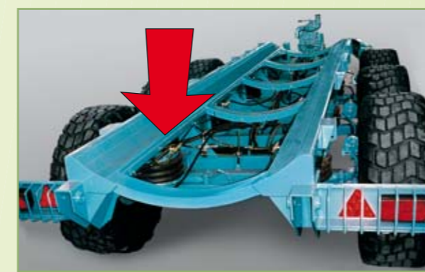
Telaio e sospensioni ad aria autolivellanti (Torpress).
